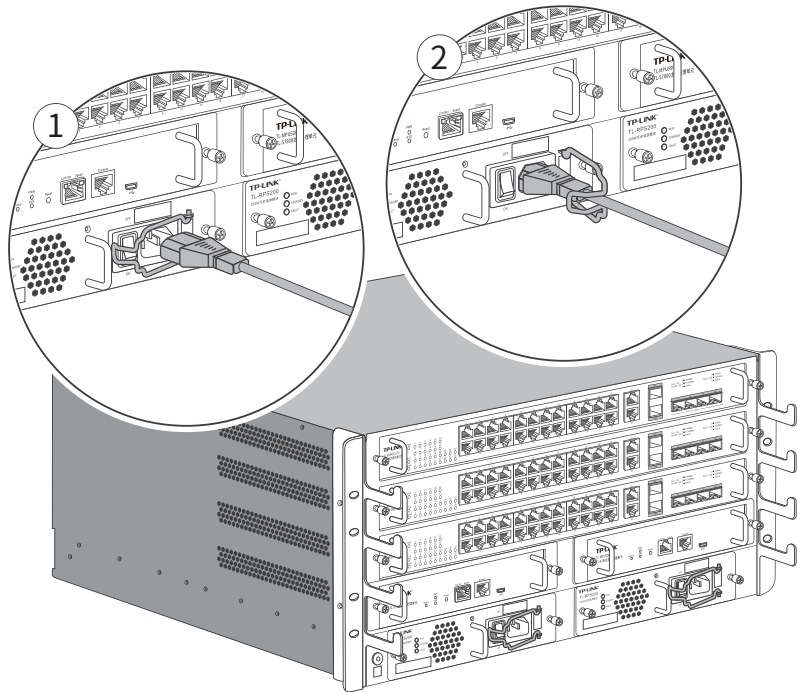
图3-2 连接电源线示意图
