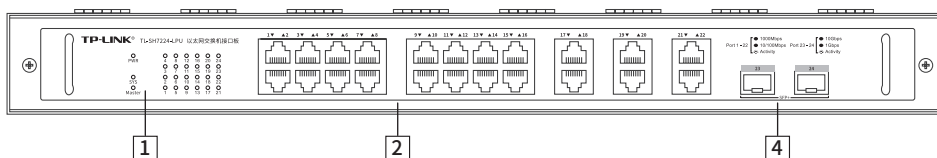
图1-9 TL-SH7224-LPU结构示意图
